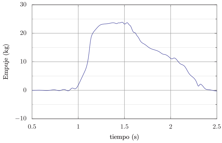
Ensayo Motor MX001
